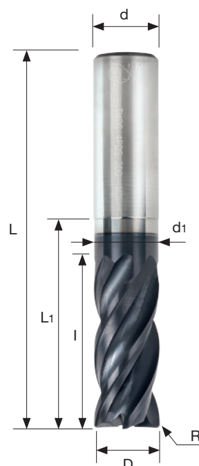
DIN 6535HB
