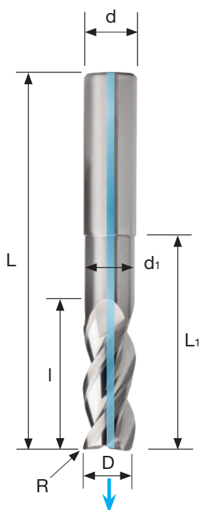
DIN 6535A
